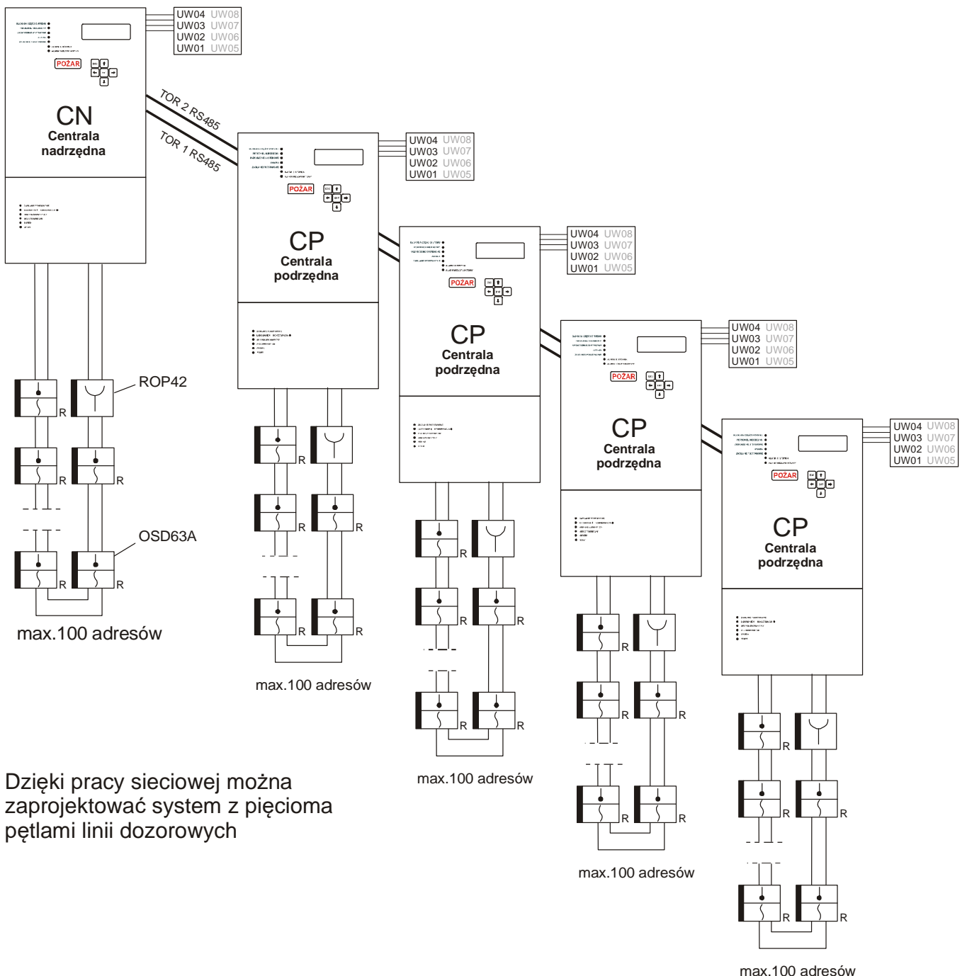
Rys. 2. System AFS42 z czterema centralami podrzędnymi
