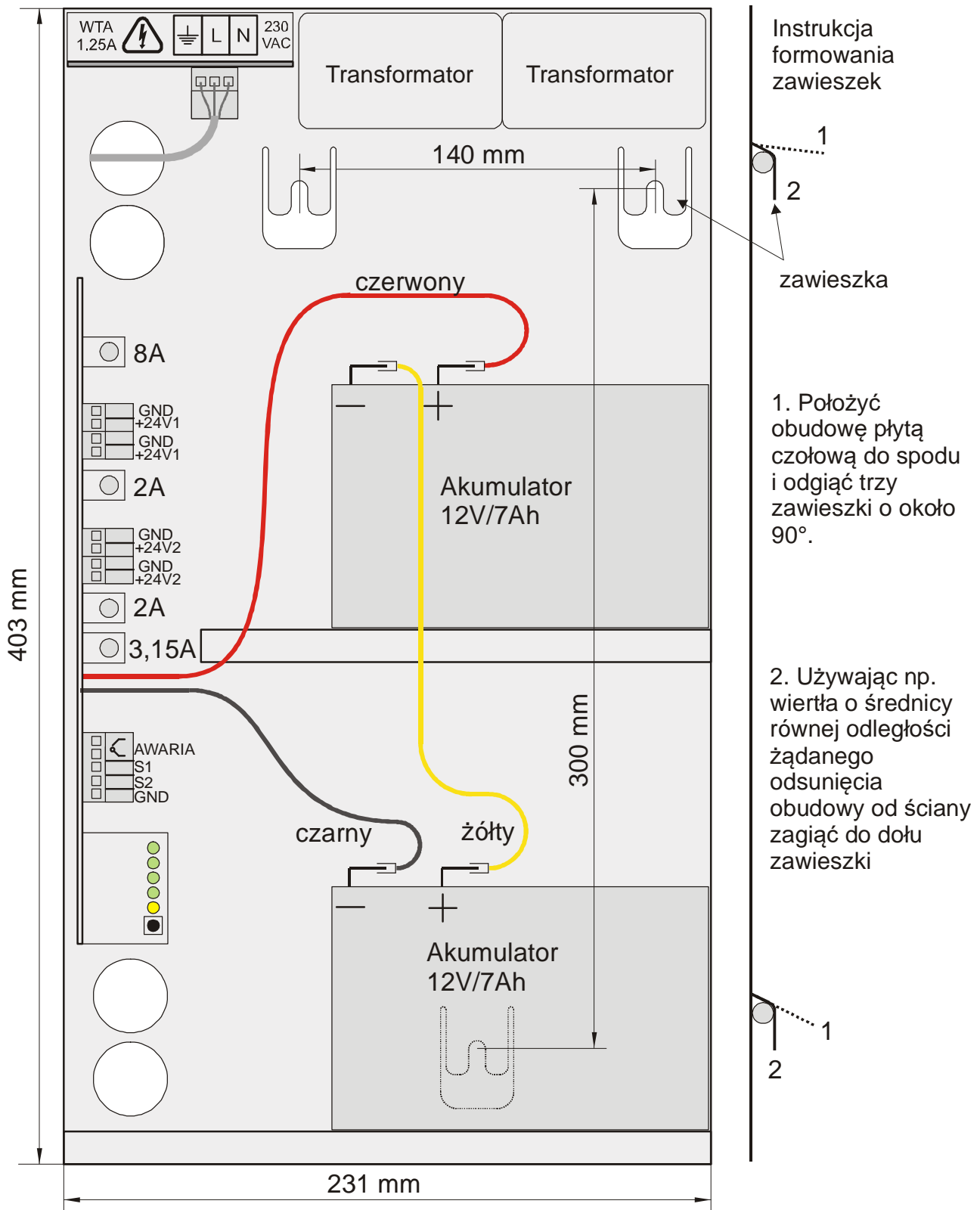
Rys. 6. Moduł zasilacza ZBP41.
