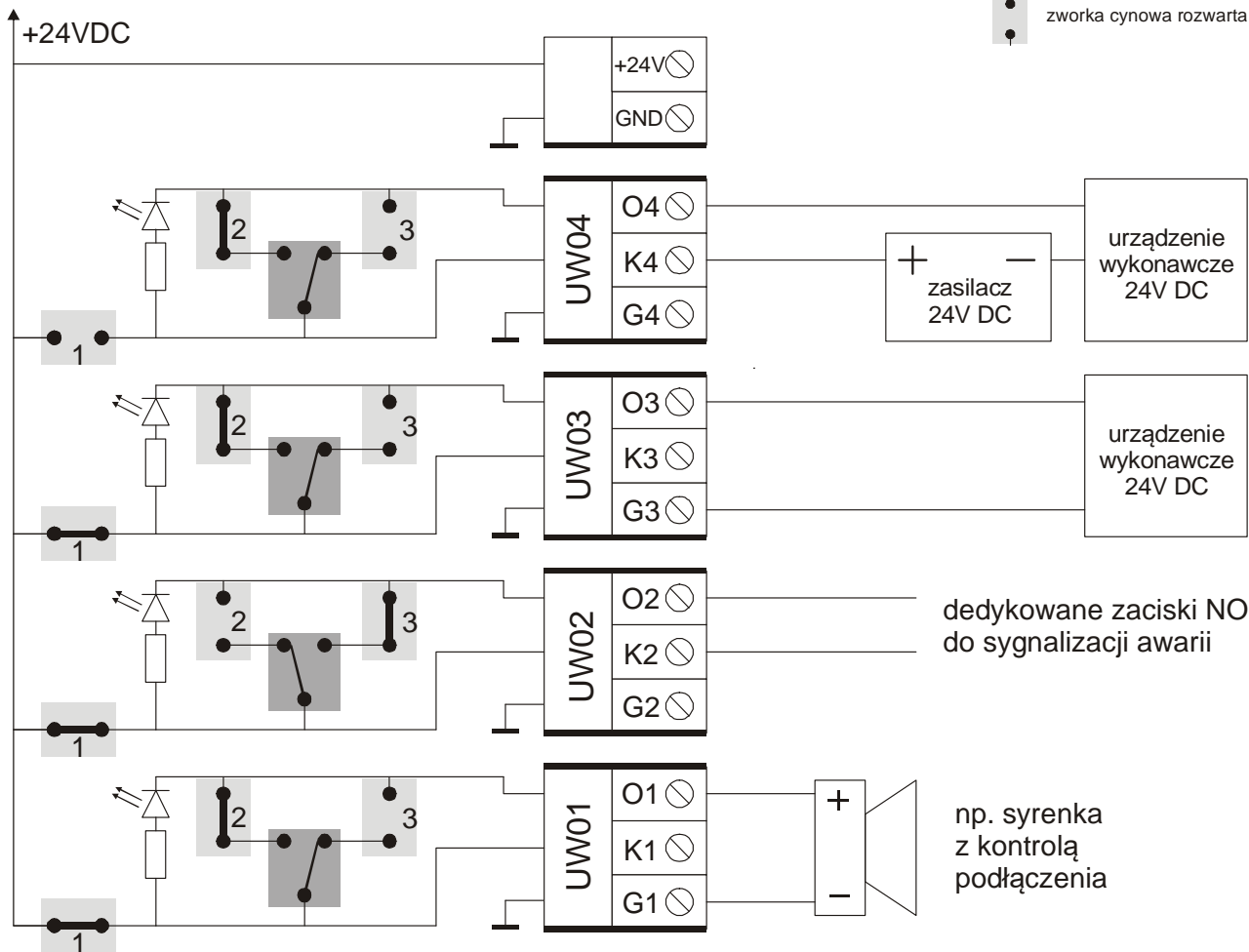
Rys. 7 Rozmieszczenie i funkcje zacisków do podłączenia UW
