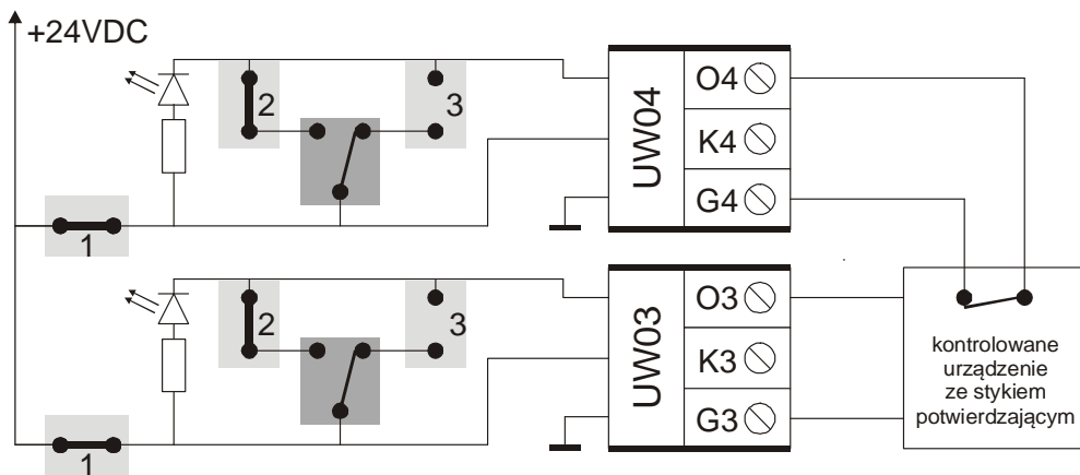
Rys. 7b Przykład "Wejście (kontrola załączenia UW)"
